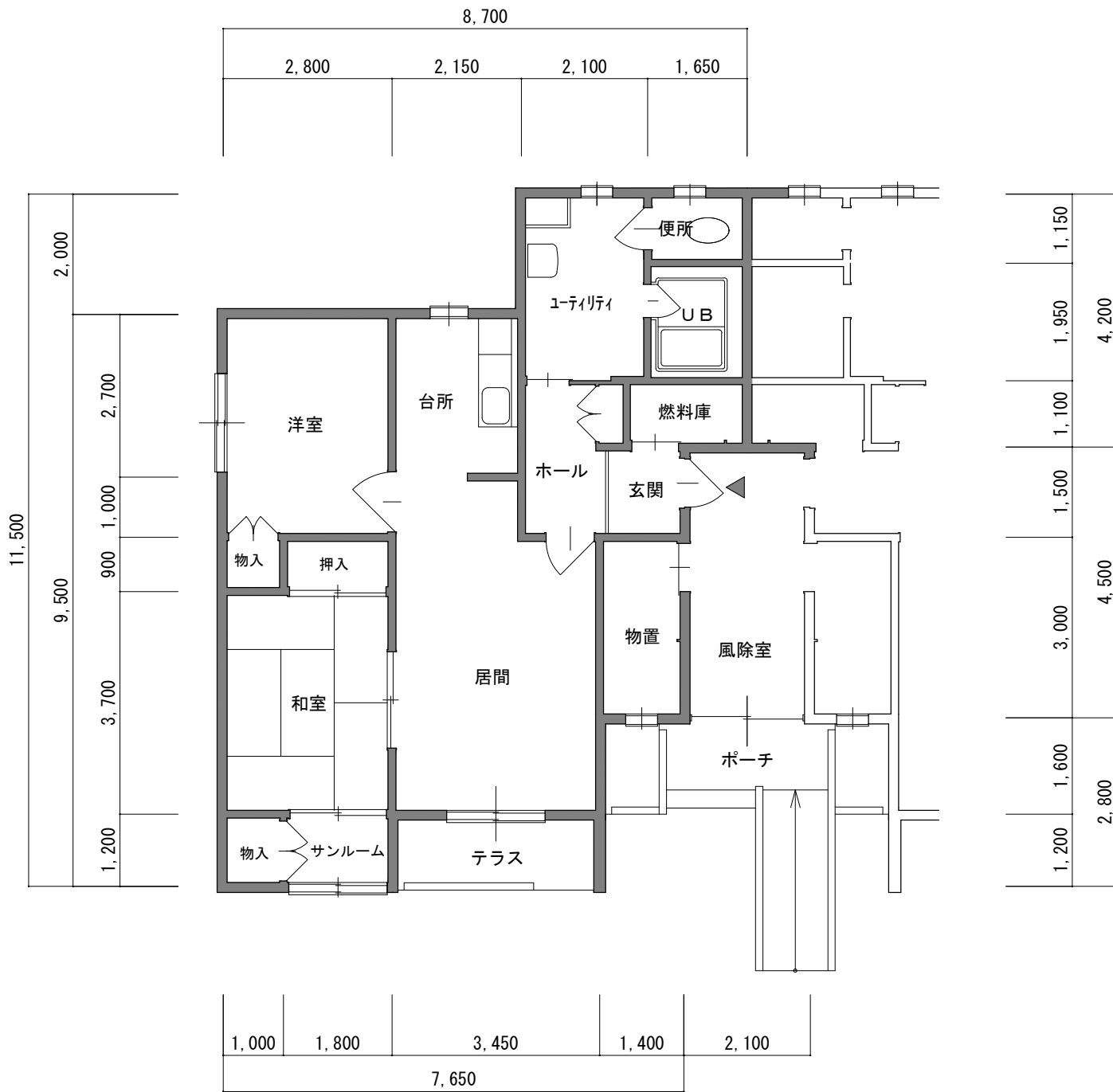
川添2LDK (H8) もみじ
